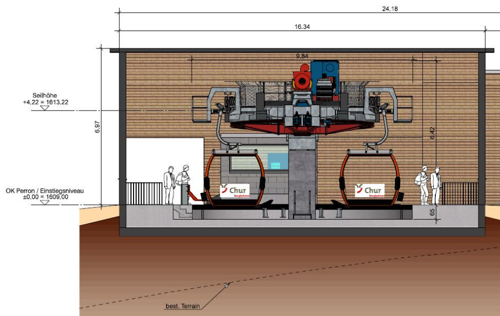
Abb. 24 Beispiel Querschnitt einer Bergstation
